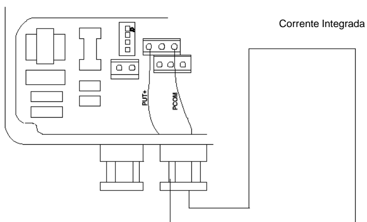
Figura 7.4 (c) Conexão do Contador Eletrônico
