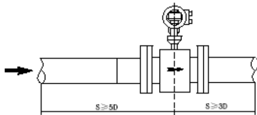
Figura A (Tubo horizontal) Requisitos do trecho reto do tubo da parte anterior e posterior
