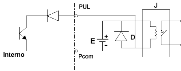
Figura 7.5 (c) Ligação da saída de pulso digital com rele
