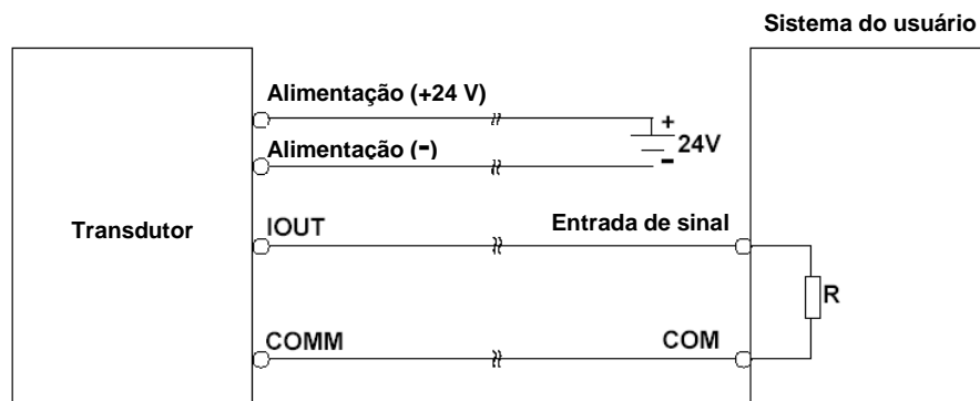
Figura 7.6 (c) Ligação a Quatro Fios
