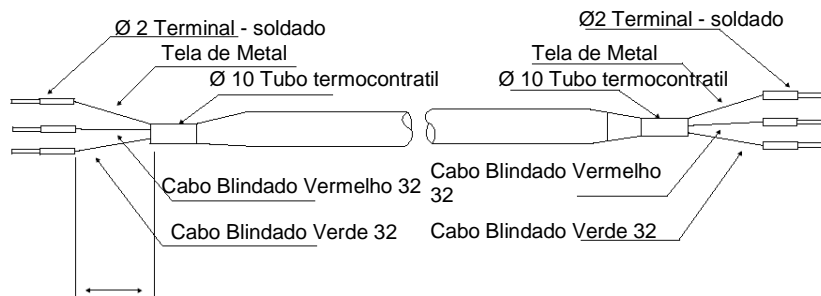
Figura 7.3 (b) Conexão e Etiquetas de linhas de Sinal do medidor quadrado
