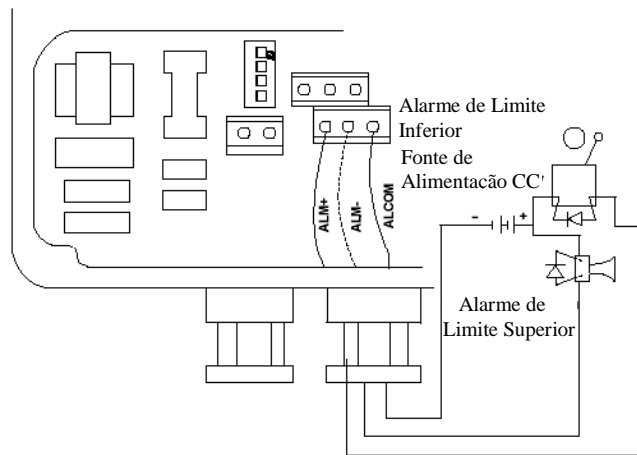
Figura 7.4 (d) Conexão de Saída de Alarme
