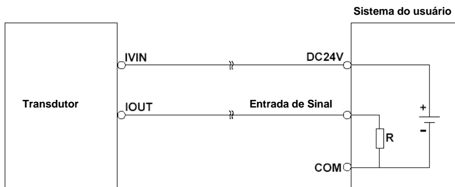
Figura 7.6 (a) Ligação a dois fios
