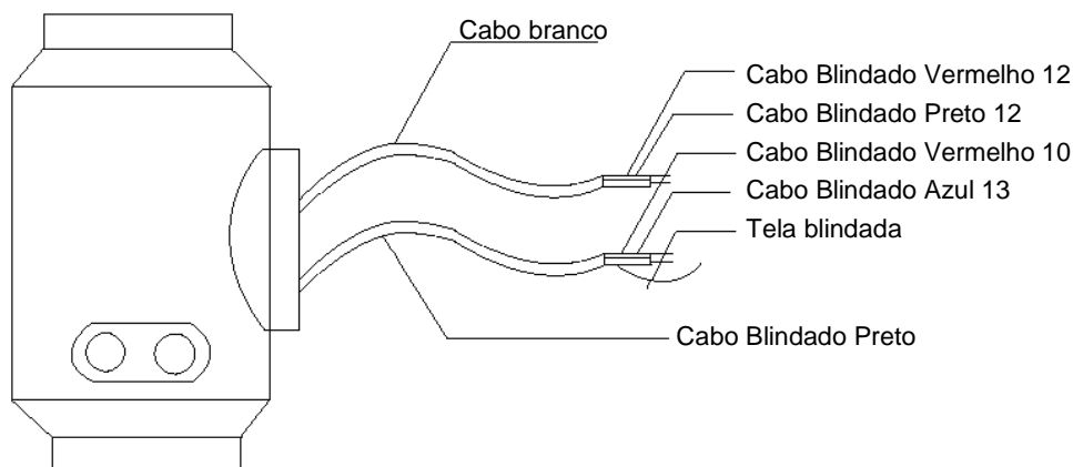
Figura 7.3 (d) Disposição e marcação da linha de sinal de medidor redondo
