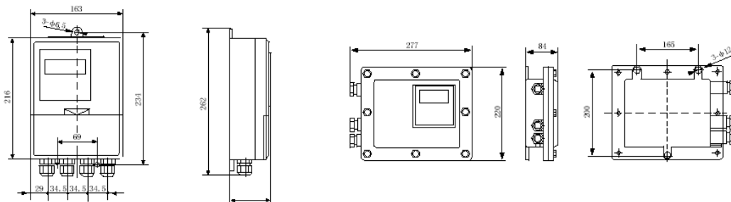
Transdutor do Tipo Remoto Normal
