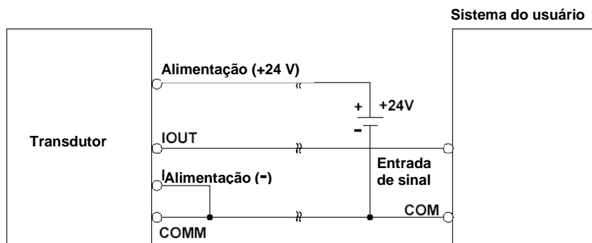
Figura 7.6 (b) Ligação a três fios
