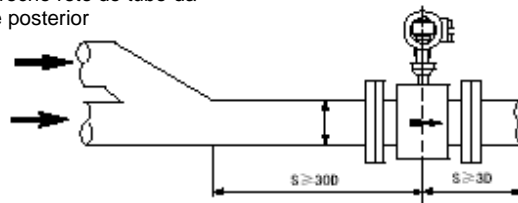
Figura G (Líquido misturado) Requisitos do trecho reto do tubo da parte anterior e posterior
