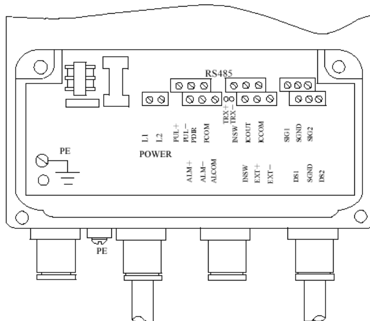
Figura 7.3 (a) Diagrama de fiação do Medidor Quadrado
