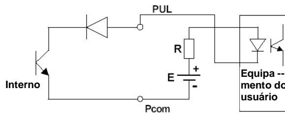
Figura 7.5 (b) Ligação da saída de pulso digital com foto-aclopador
