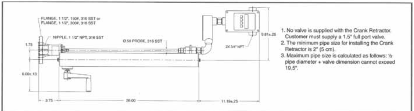
Figura 7: Montagem com manivela retrátil para alta pressão ROSCA NPT 600 psi g, Flange ANSI 150# e ANSI 300#
