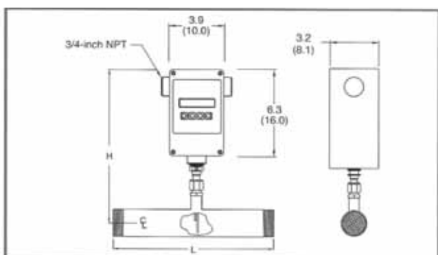
Figura 5: Invólucro Remoto
