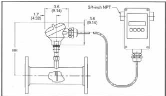
Figura 5: Invólucro Remoto
