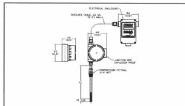
Figura 5A: Sensor
