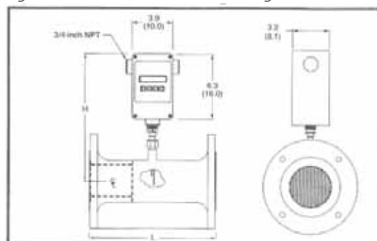
Figura 2: em Linha de 1/2" a 6" - Flanges 150#
